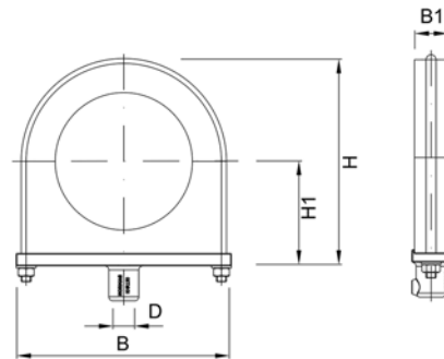
KHR.../ KHRS...pipe supports
