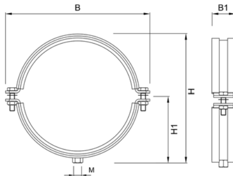
KPC.../ KPCS...pipe clamps
