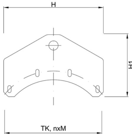
KLL... Lifting lug
